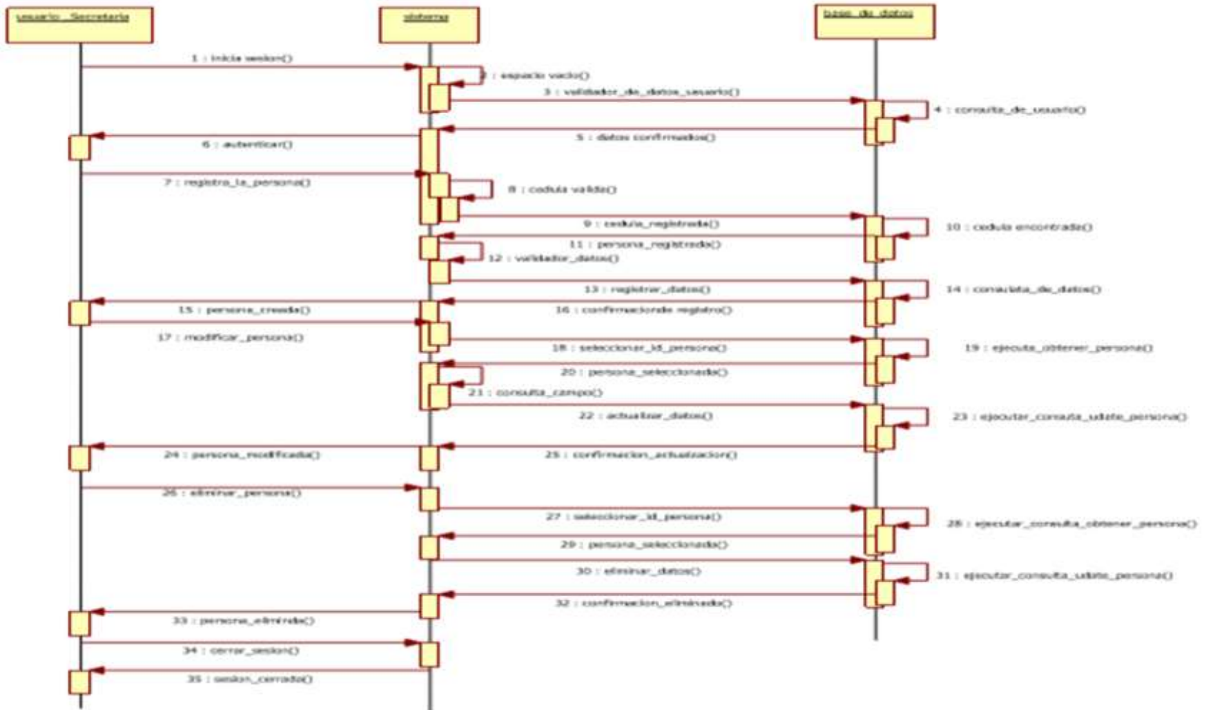
Figura 20: Diagrama Sistemas
