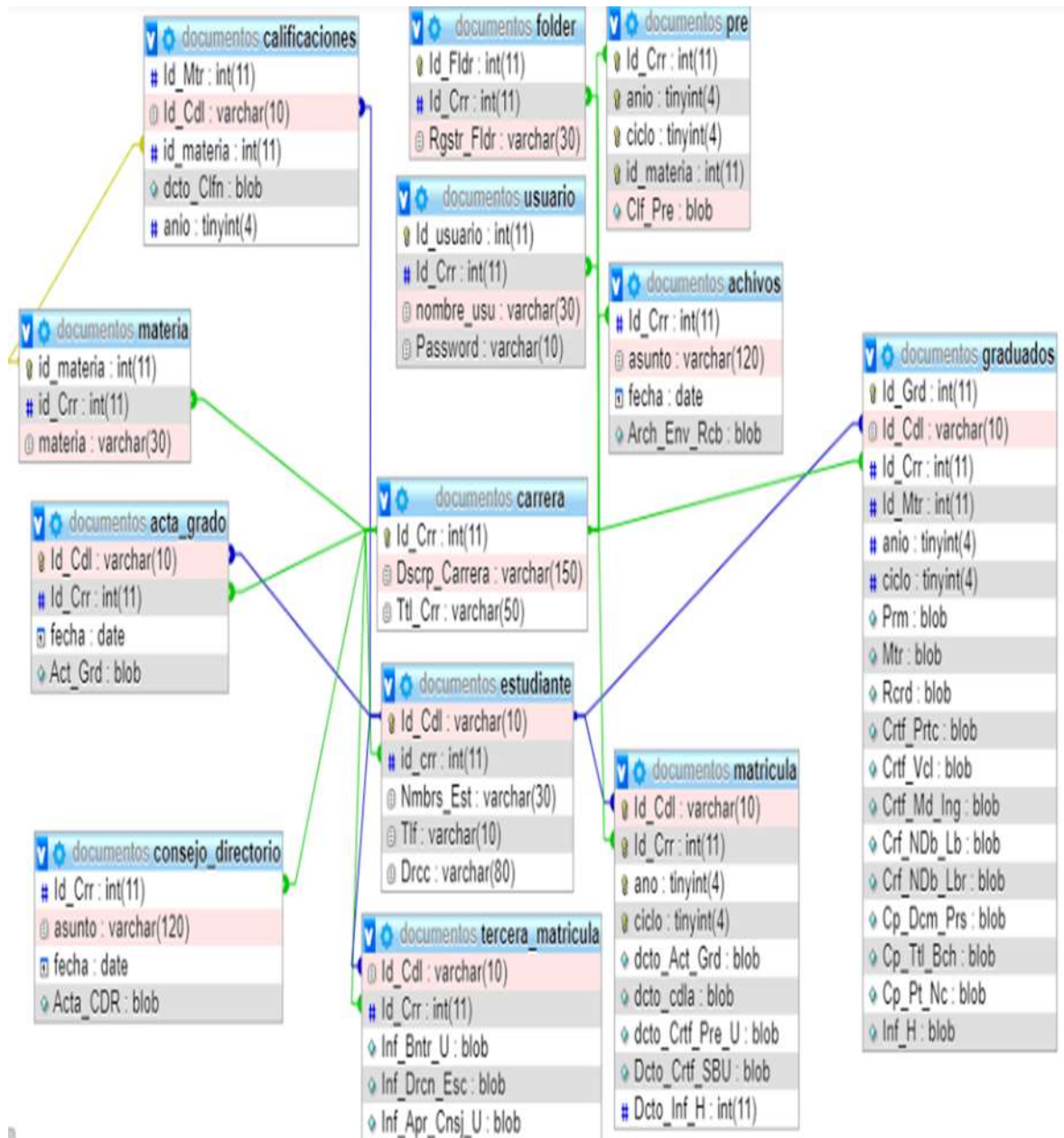
Figura 12: Entidad Relación
