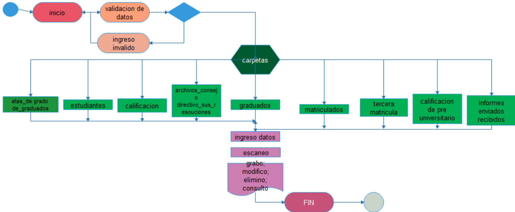
Figura 21: Diagrama Actividades
